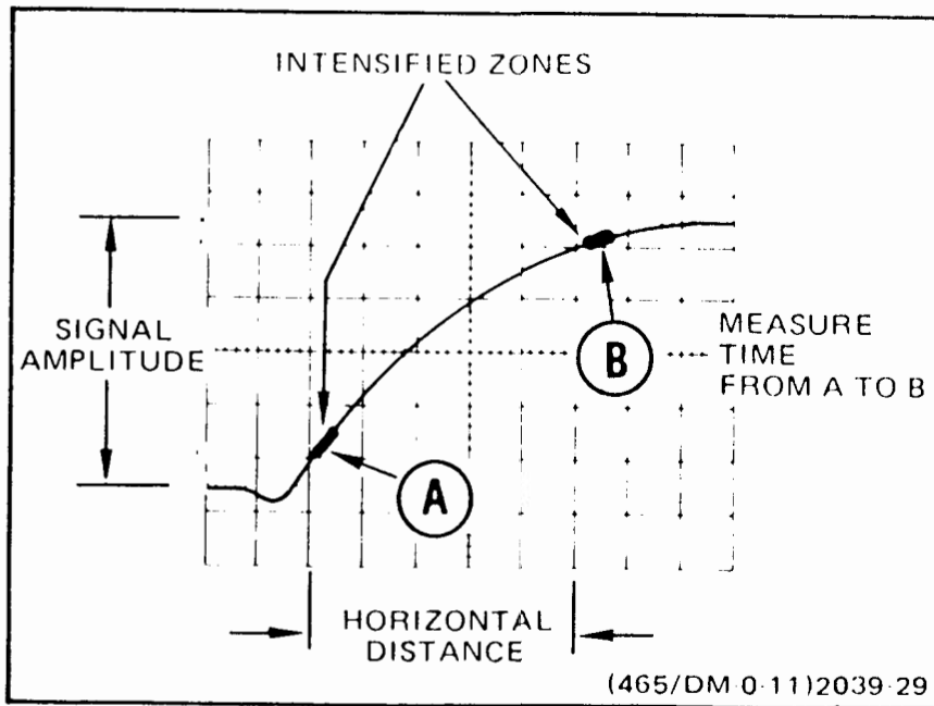
Fig. 28. Risetime.
