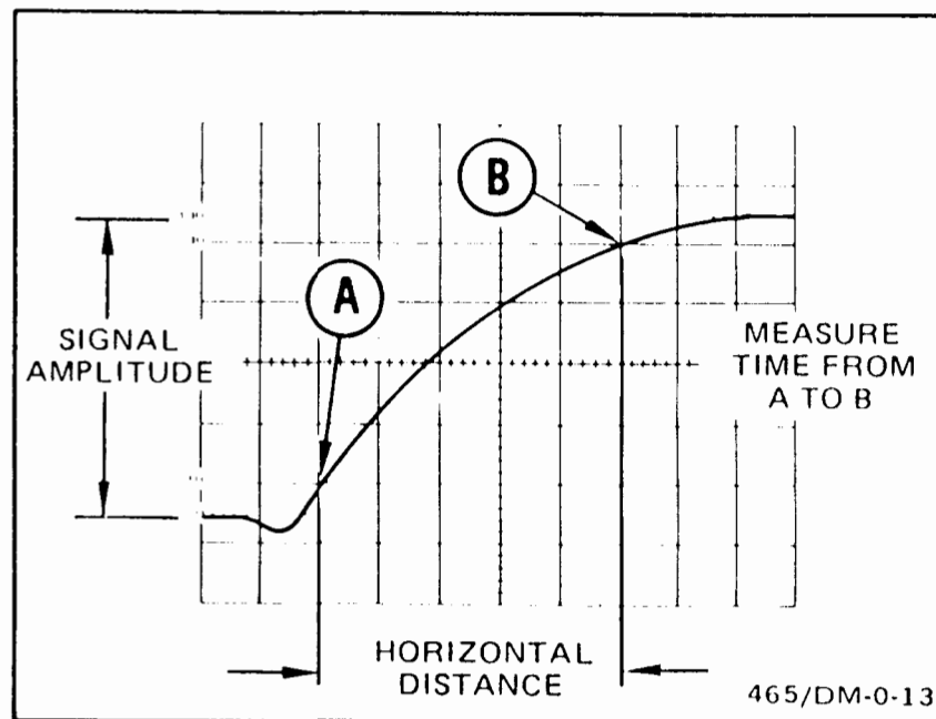
Fig. 19. Risetime.
