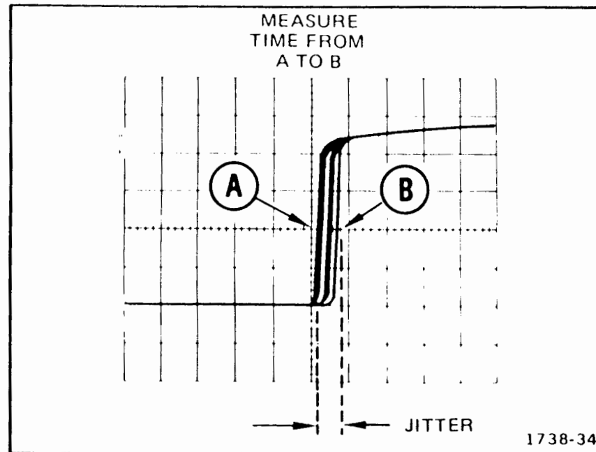
Fig. 23. Pulse jitter.
